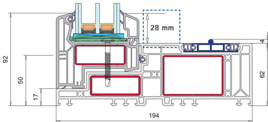
Innenansichtshöhe des Festflügels: 28 mm
